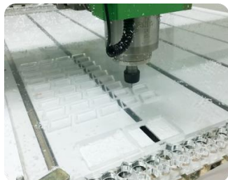
ЧПУ станки для точного криволинейного раскроя листовых пластиков
